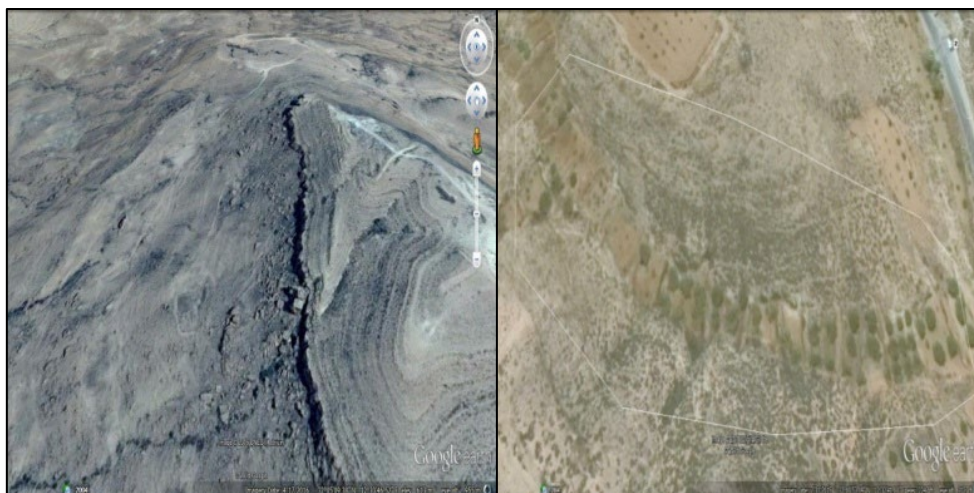
شكل 1: صور جوية مكان جمع المستخلصات النباتية من منطقة يفرن عبر خرائط google، خط طول 32.09 0 وخط عرض 12.51 0 .
